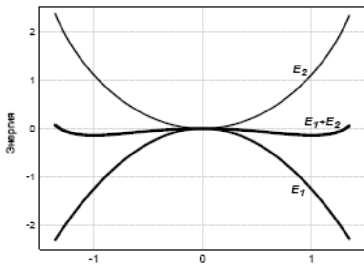
Рис. 1. Графики функции энергии E_1 + E_2 и ее компонент E_1 и E_2 в сечении x_1 + x_2 .
