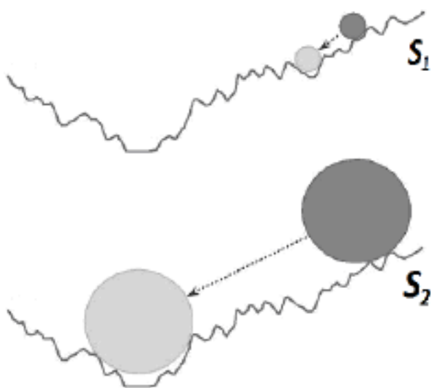
Рис. 3. Эффект сглаживания когнитивного энергетического ландшафта: S_1 < S_2 .
