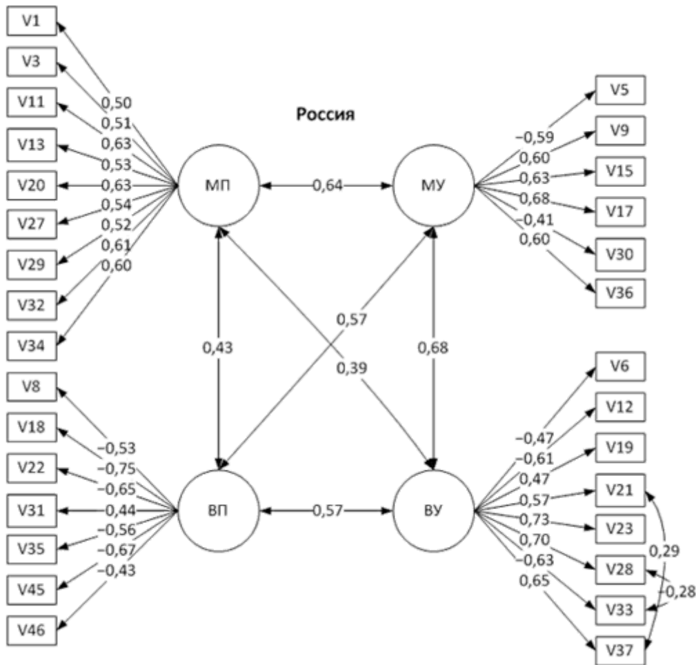
Рис 1. Параметры модели RU-2.
